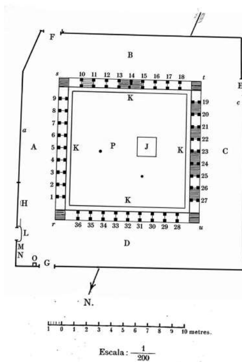
Planta del claustre (croquis per don Ramon Arabia i Solanas).
